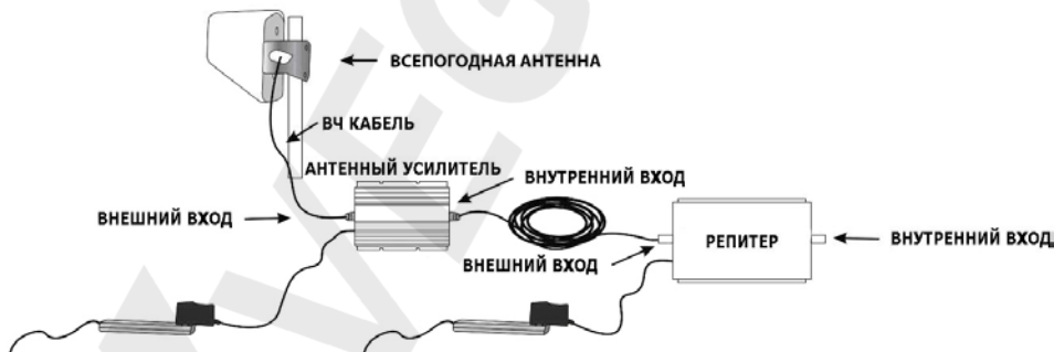
Схема подключения усилителя антенного
