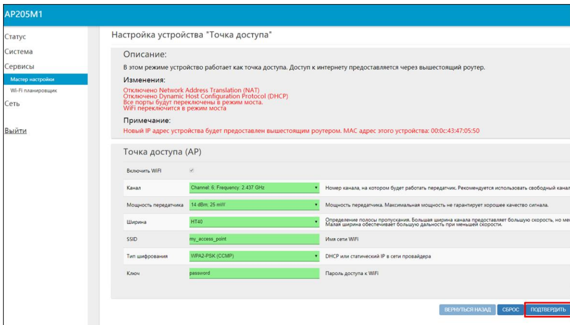
Рисунок 2.7.3 – Проверка введенных данных
