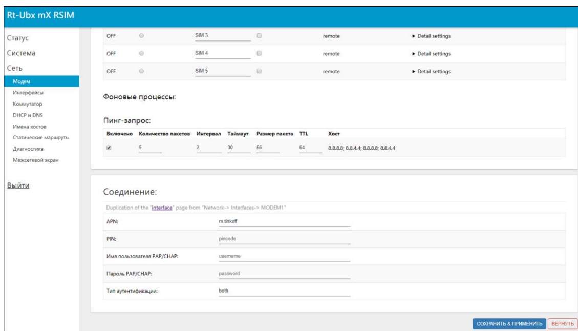
Рисунок 5.8.4 – Информация о настройках подключения активной SIM-карты
