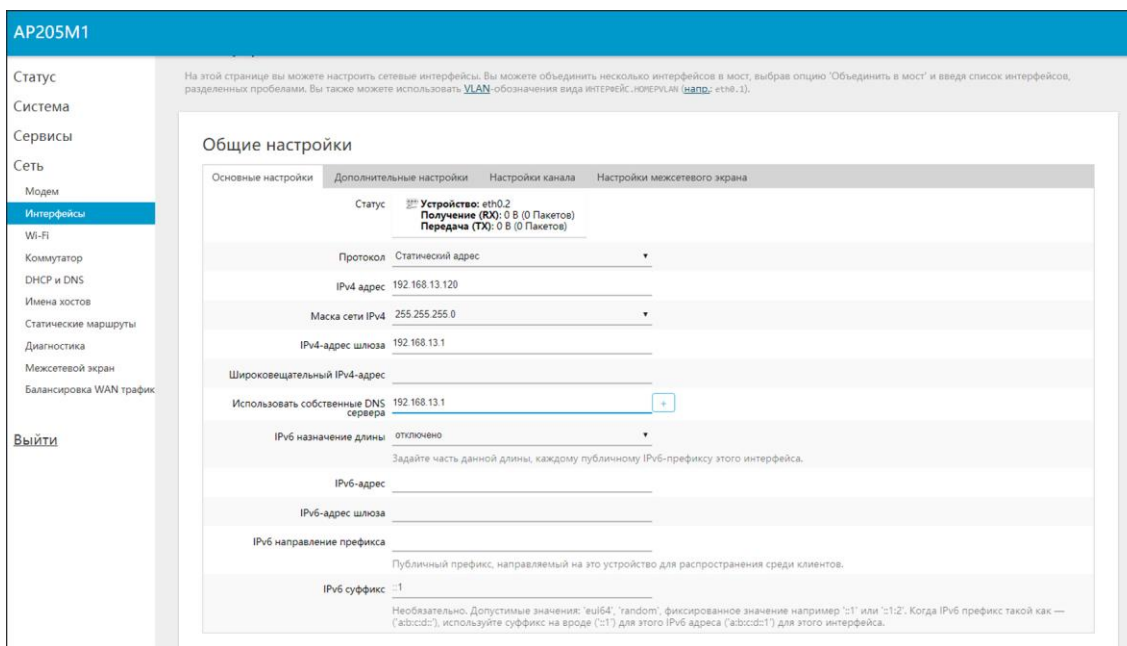
Рисунок 3.3.9 – Основные настройки интерфейса lan со статическим IP-адресом
