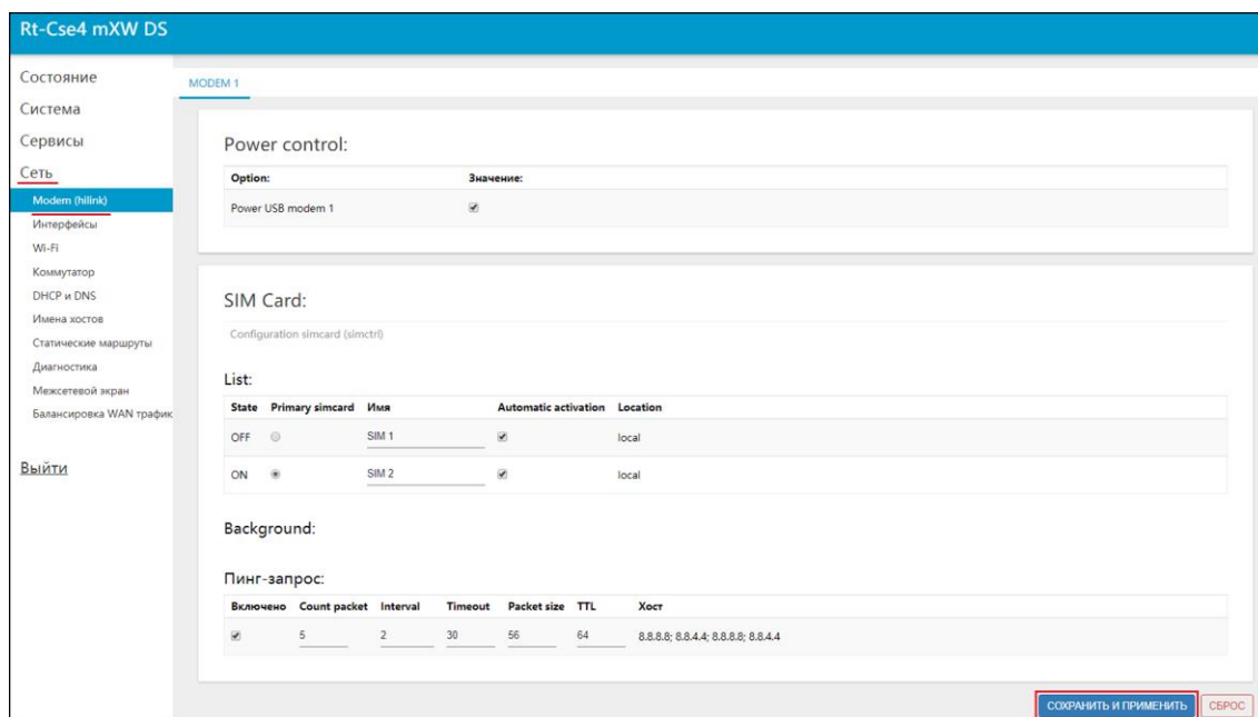
Рисунок 5.7.1 – Настройка работы модема с SIM-картами
