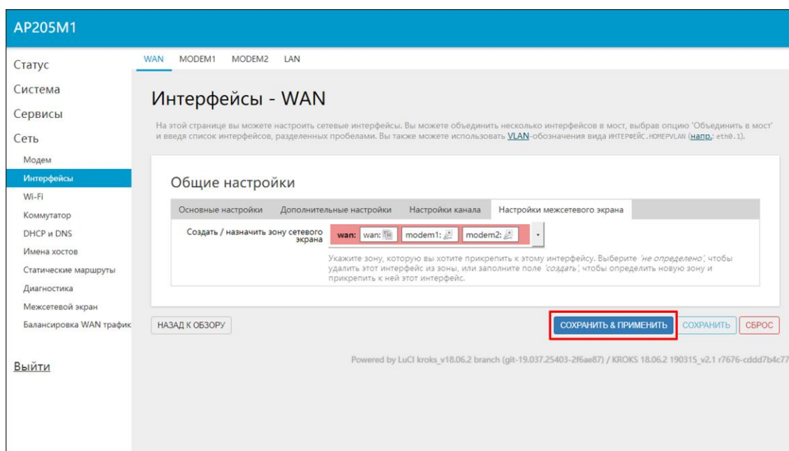
Рисунок 3.4.12 – Настройка зоны межсетевое экрана
