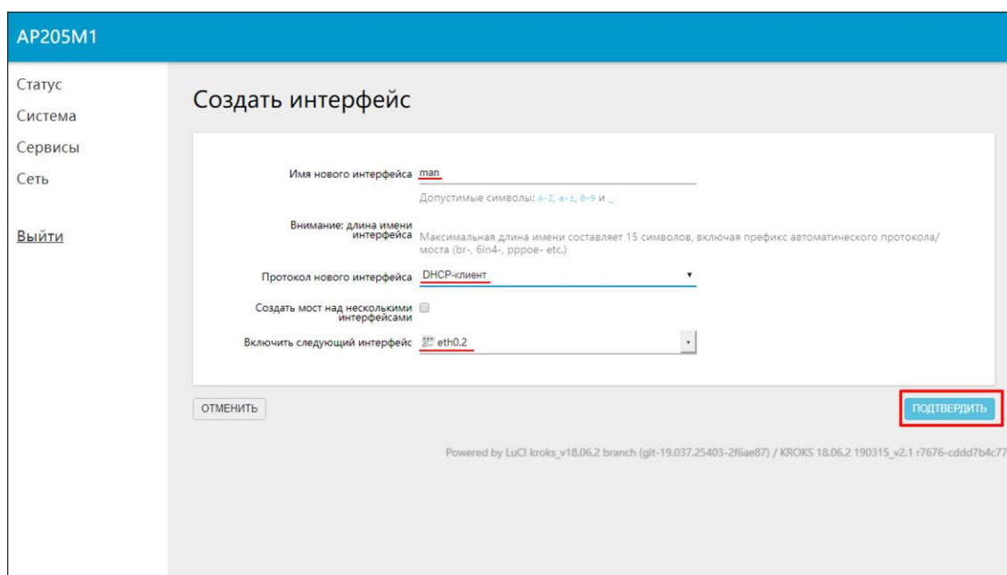
Рисунок 3.4.8 – Создание интерфейса man с динамическим IP-адресом
