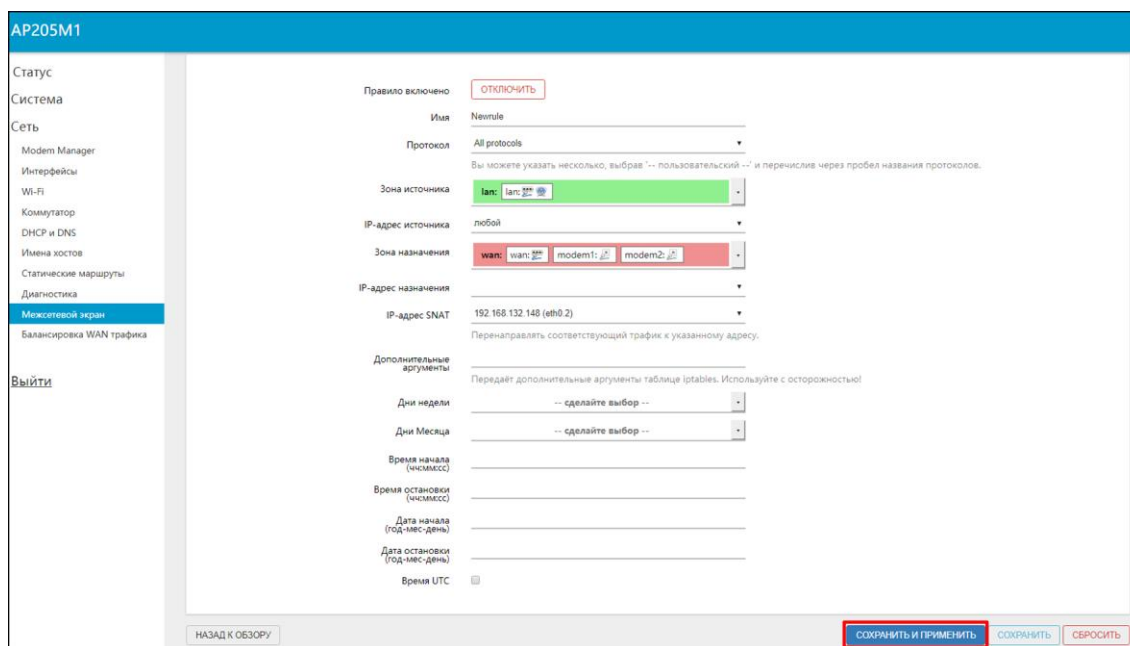
Рисунок 7.3.3 – Расширенные настройки правила использующего метод SNAT
