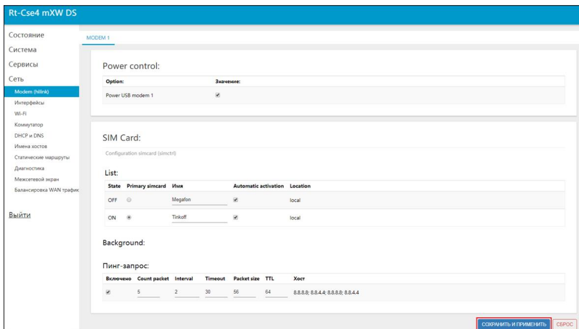
Рисунок 5.7.2 – Настройка основного и резервного каналов связи с 3G/4G оператором
