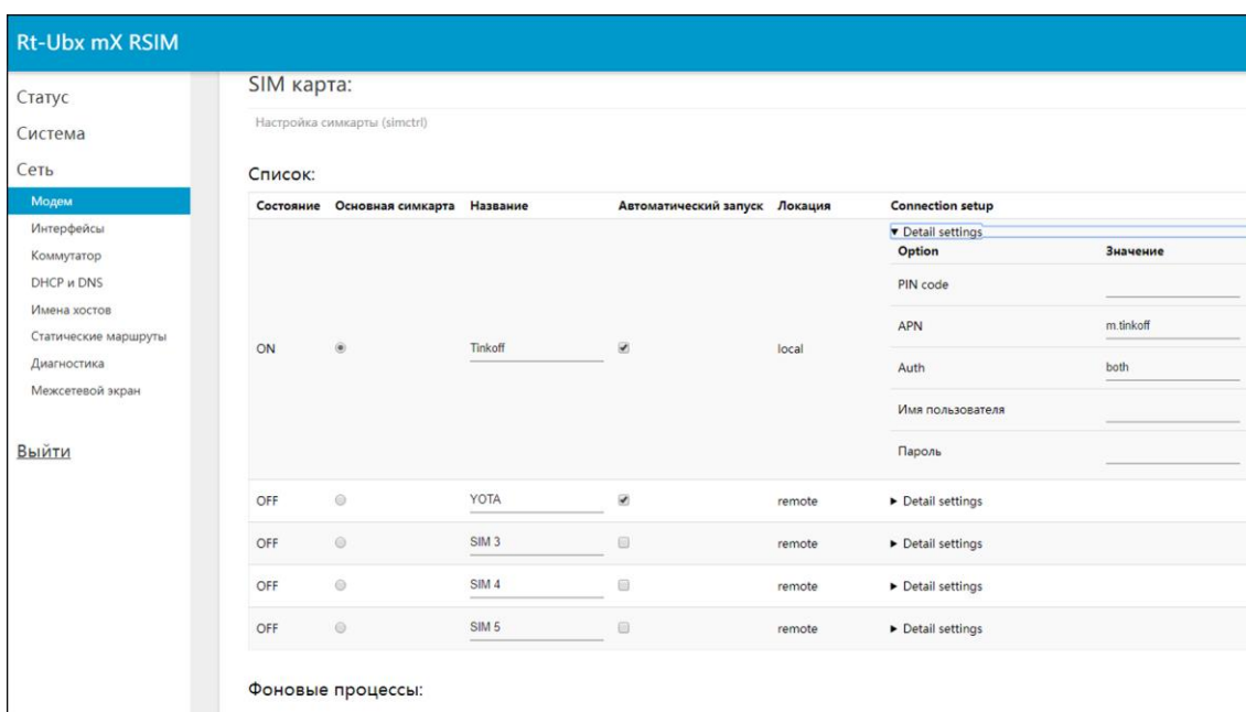
Рисунок 5.8.3 – Настройки соединения
