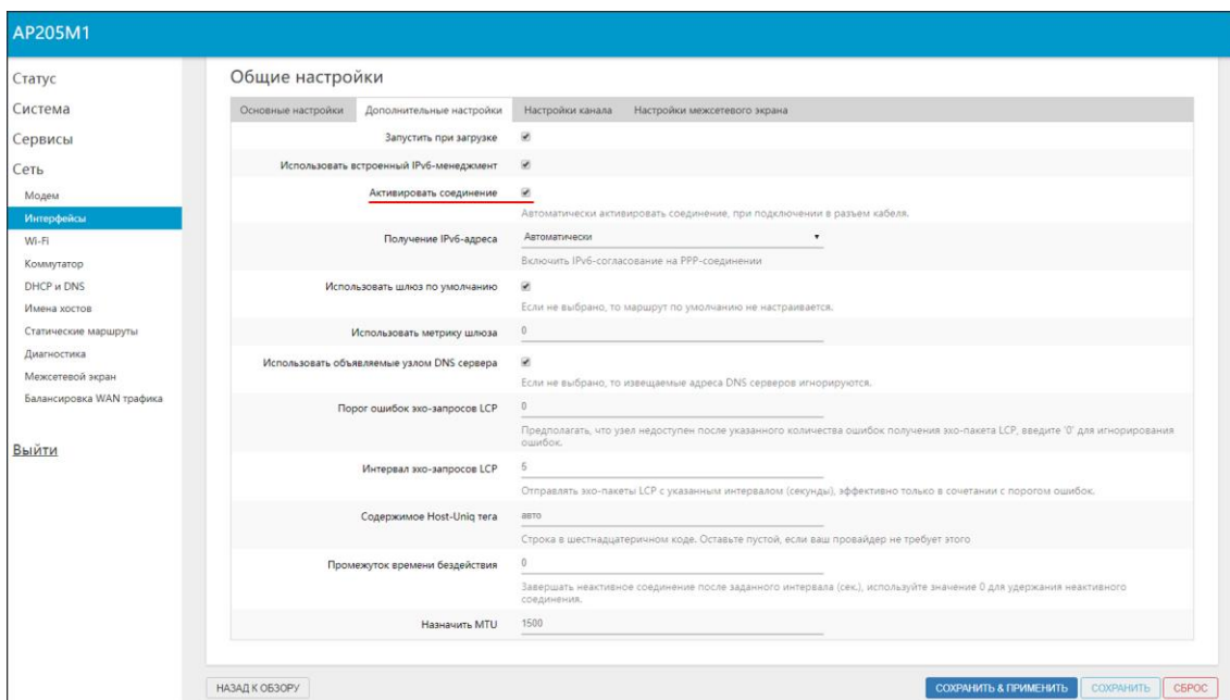
Рисунок 3.5.4 – Дополнительные настройки соединения по протоколу PPPoE
