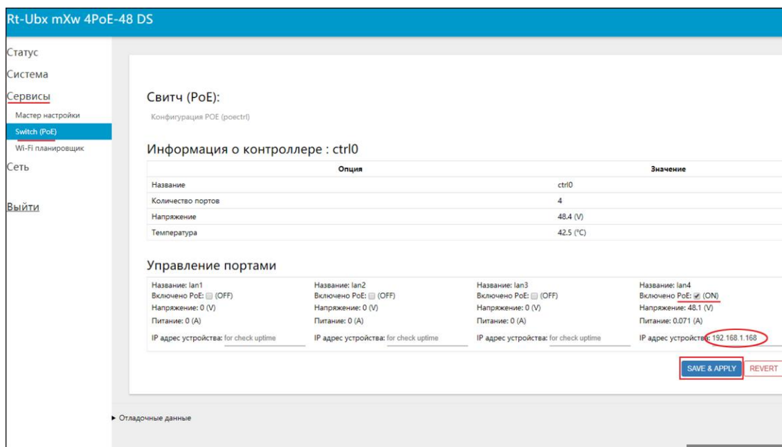
Рисунок 4.4.1 – Управление PoE питанием портов
