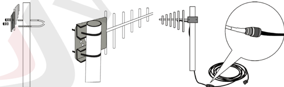
Пример установки всепогодной антенны типа «волновой канал» (антенна Яги)
