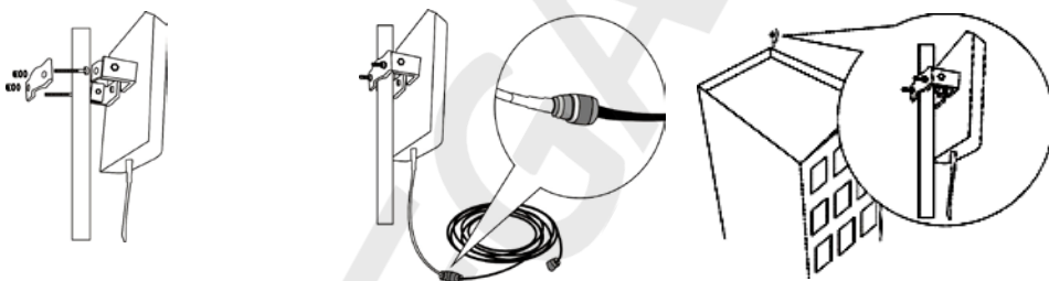
Пример установки всепогодной панельной антенны
