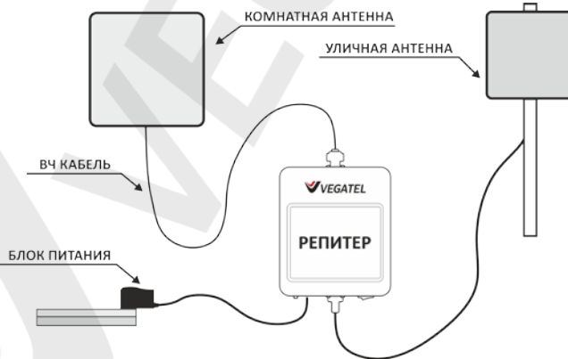
СХЕМА ПОДКЛЮЧЕНИЯ РЕПИТЕРА
