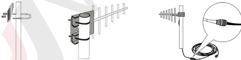
Пример установки всепогодной антенны типа «волновой канал» (антенна Яги)
